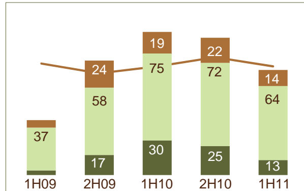
Zircon (kt)
