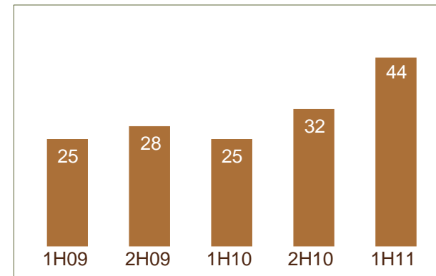
Pigment (kt)
