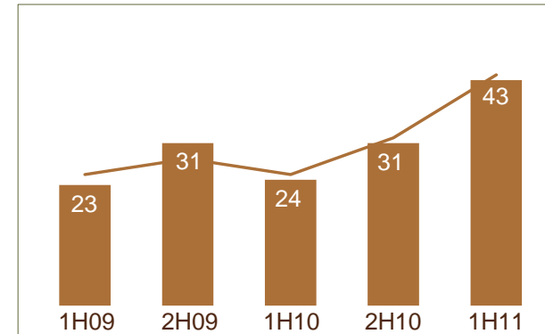
Pigment (kt)
