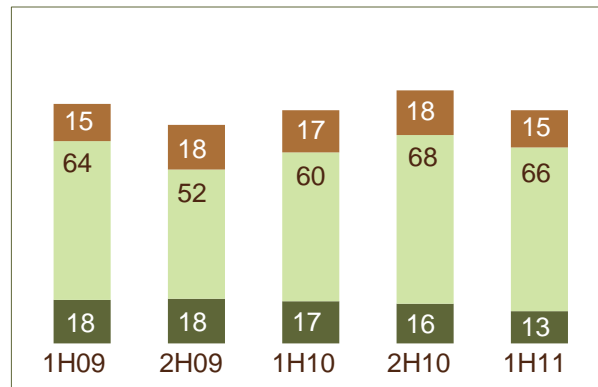
Zircon (kt)
